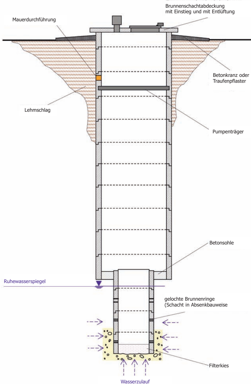
Abb. 3: Schachtbrunnen mit Betonfertigteilen © Martin Bachner – Handbuch für Brunnenbesitzer
